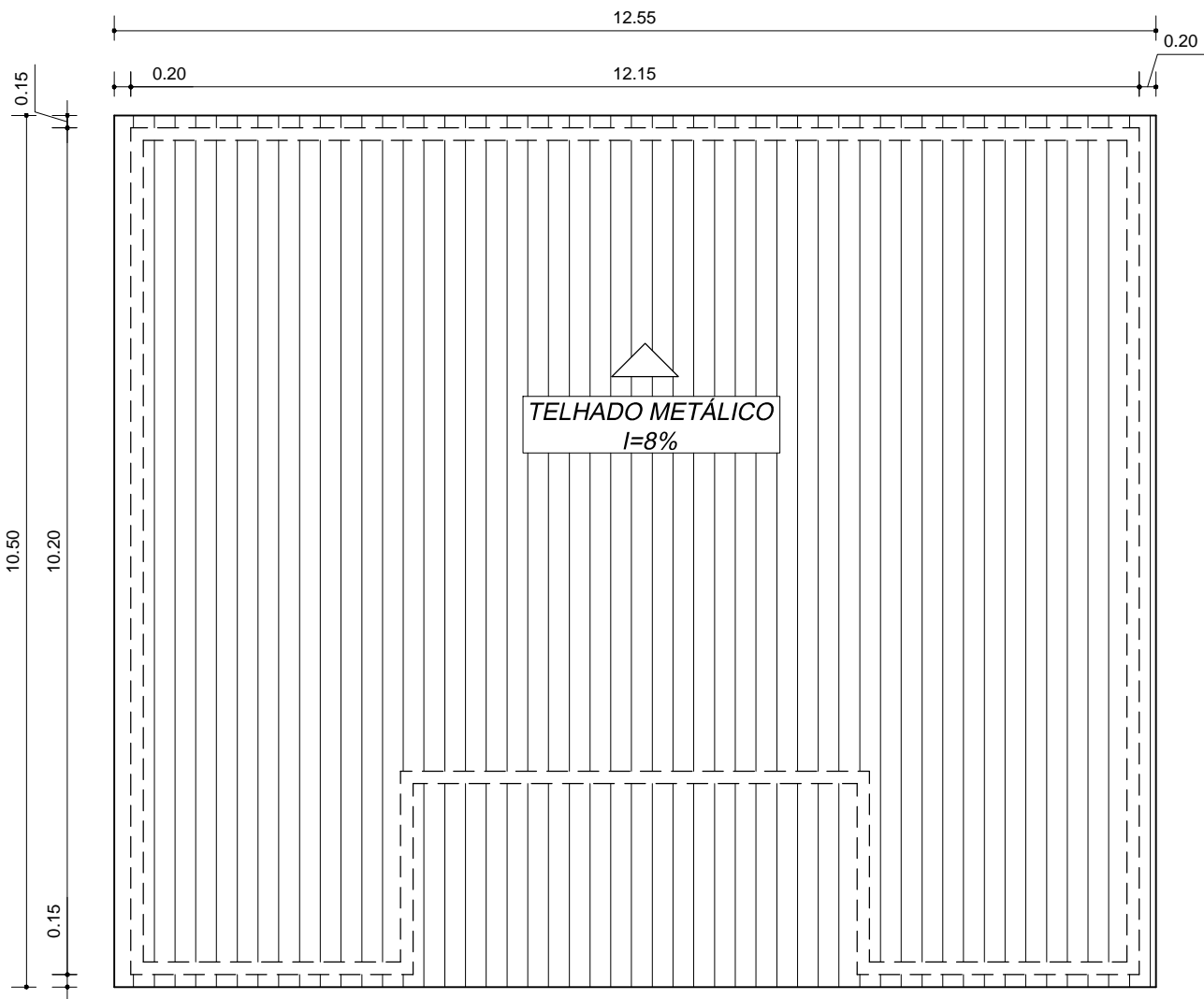
PLANTA DE COBERTURA ESC:1/75
