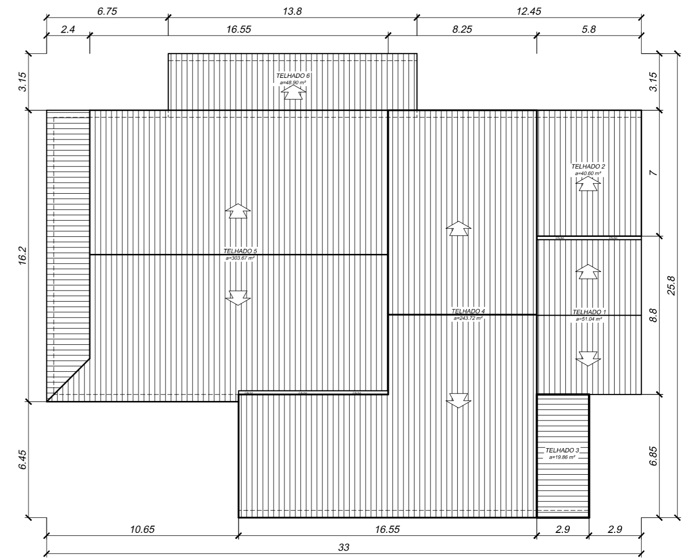
PLANTA BAIXA - BRAÇO DO SUL ESC.:1/200
