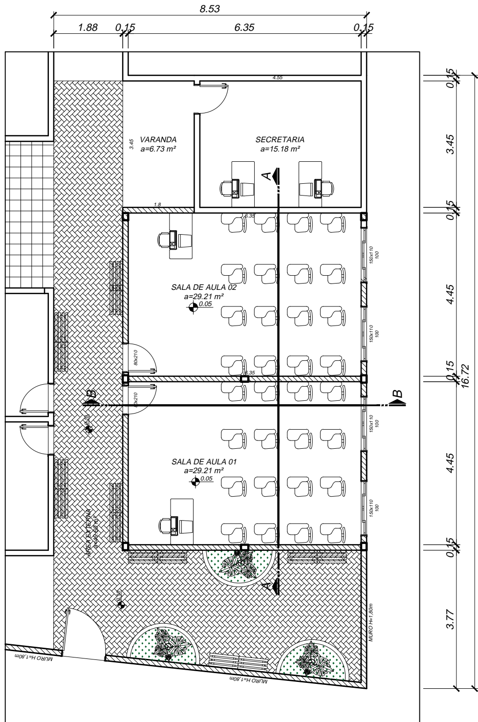
PLANTA BAIXA - AMPLIAÇÃO ESC.: 1/100
