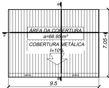
COBERTURA ESC.: 1/200
