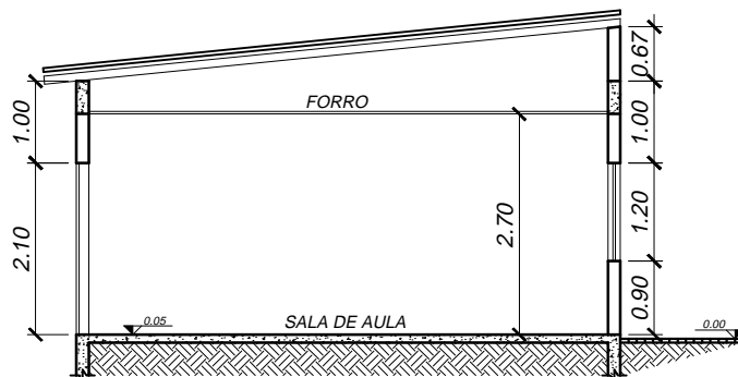
CORTE BB ESC.: 1/100
